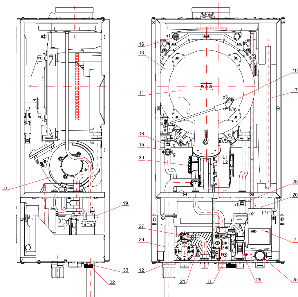
Rys. 2.2.1.1. Rozłożenie elementów w kotle ECOCONDENS NEX dwufunkcyjnym
