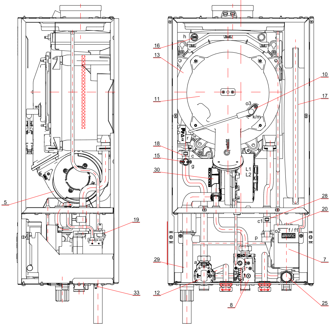
Rys. 2.2.1.2. Rozłożenie elementów w kotle ECOCONDENS NEX jednofunkcyjnym
