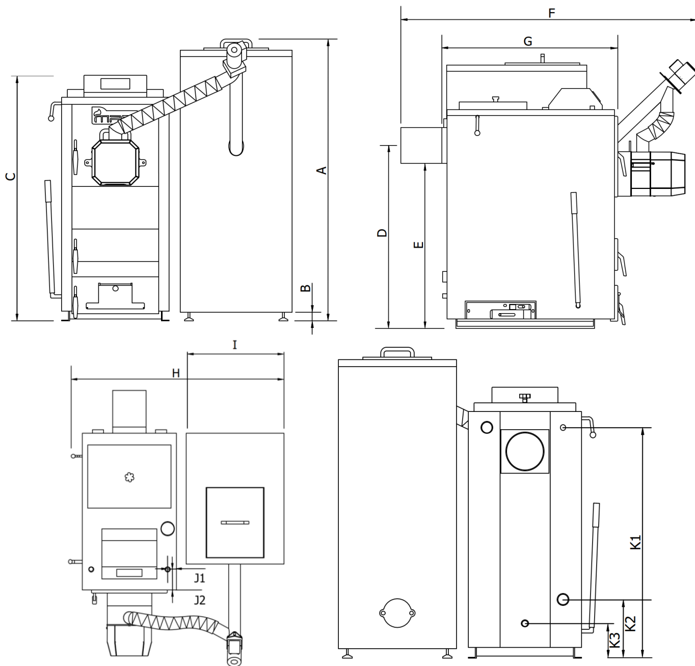
Rysunek 2. Podstawowe wymiary kotła MPM Wood Pell
