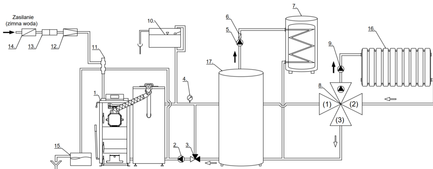
Rysunek 3. Przykładowy schemat podłączenia kotła MPM Wood Pell w układzie otwartym.
