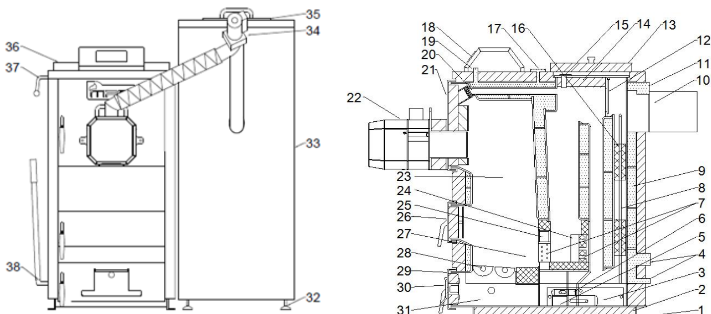
Rysunek 1. Schemat konstrukcji kotła
