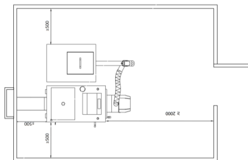
Rysunek 5. Ustawienie kotła w pomieszczeniu kotłowni.
