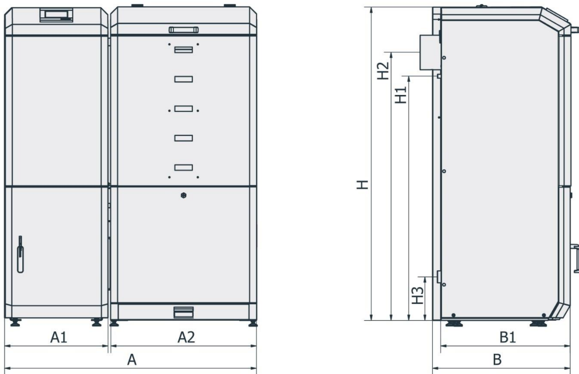
Rys. 2. Podstawowe wymiary kotła Kamen PrimaPell.
