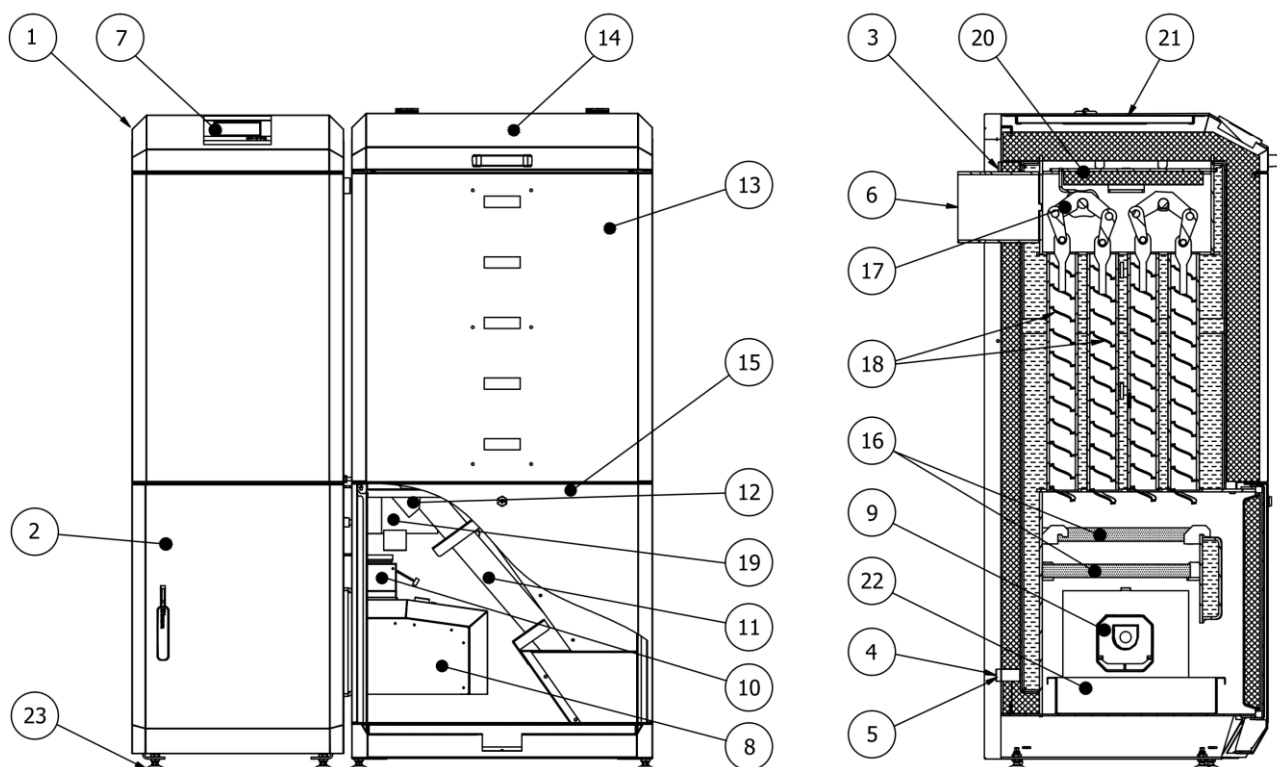
Rys 1. Schemat kotła Kamen PrimaPell (podstawowe elementy kotła + przekrój).
