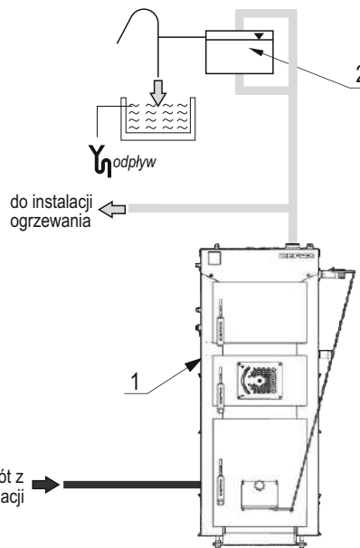
Rysunek 6. Przykładowy schemat zabezpieczeń kotła DWS w układzie otwartym: 1-kocioł; 2-otwarte naczynia wzbiorcze.
