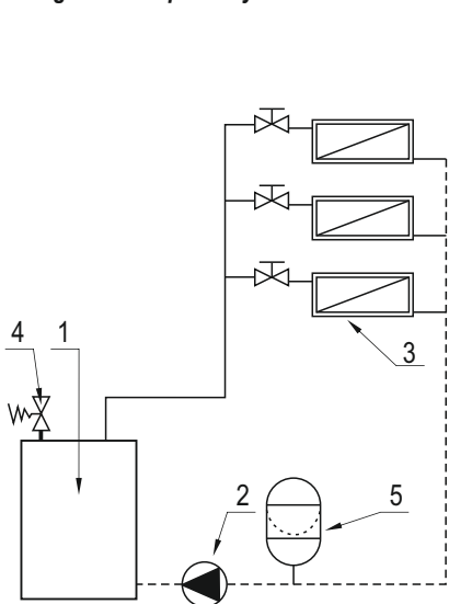
Rysunek 7. Przykładowy schemat zabezpieczeń instalacji ogrzewania wodnego wg normy PN-EN 12828: 1 - źródło ciepła; 2 - pompa obiegowa; 3 - obwód grzewczy; 4 - źródło ciepła; 5 - naczynie wzbiorcze i zalecane miejsce jego instalacji.
