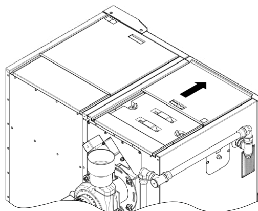
KROK 1. Przesunąć maskownicę w górnej ścianie kotła
