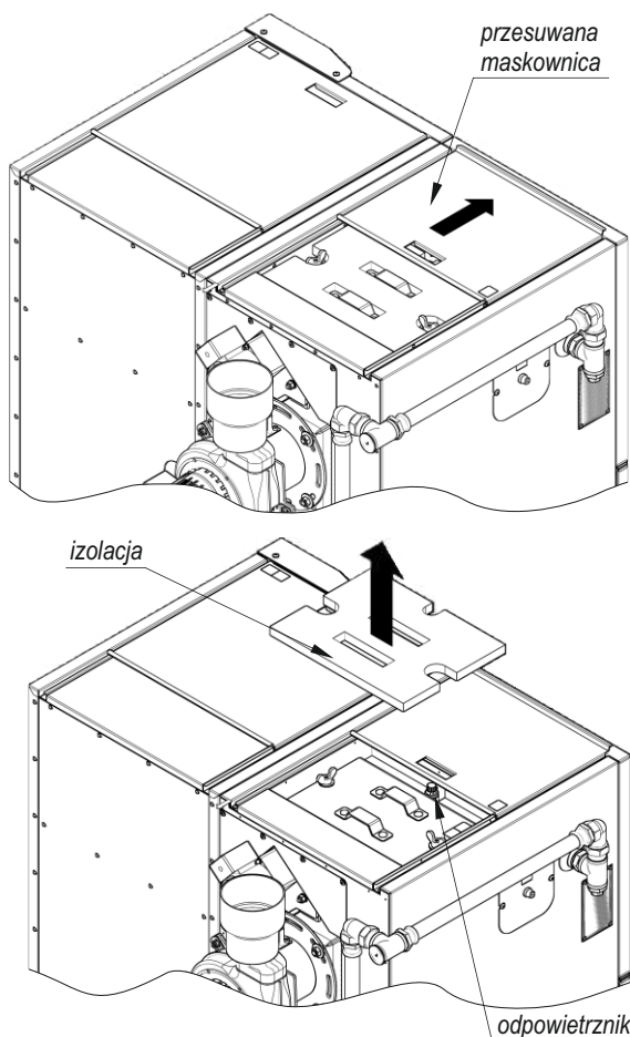
Rysunek 12. Odpowietrznik kotła.
