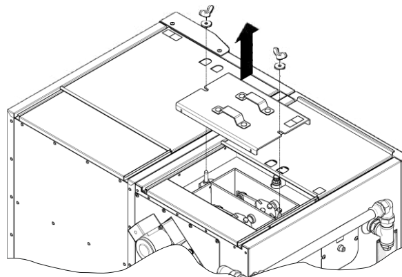
KROK 3. Odkręcić nakrętki mocujące pokrywę wyczystną, usunąć pokrywę z kotła.
