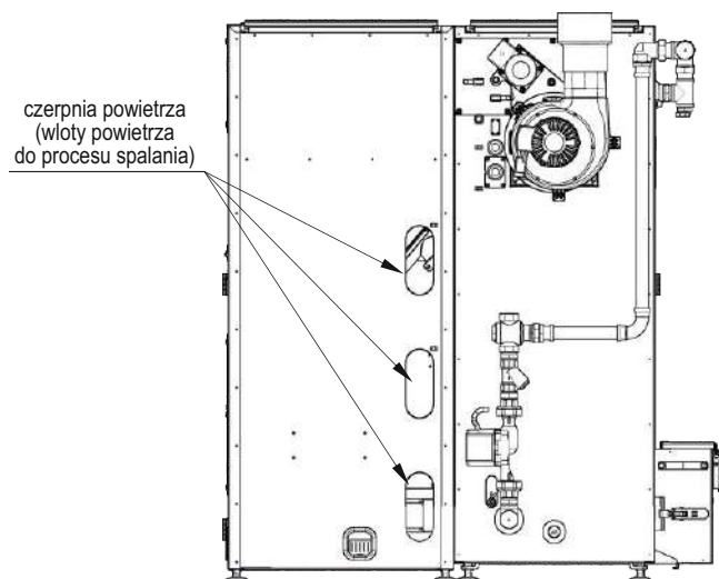
Rysunek 13. Czerpnia powietrza - otwory dolotowe powietrza
