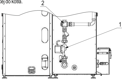
Rysunek 4. Zestaw hydrauliczny: 1-pompa obiegowa, 2-zawór termostatyczny TV 55°C.
