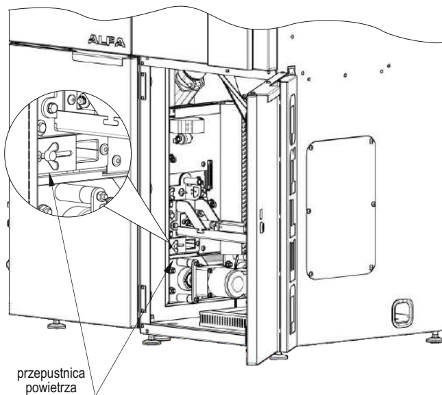
Rysunek 14. Położenie przepustnicy powietrza.
