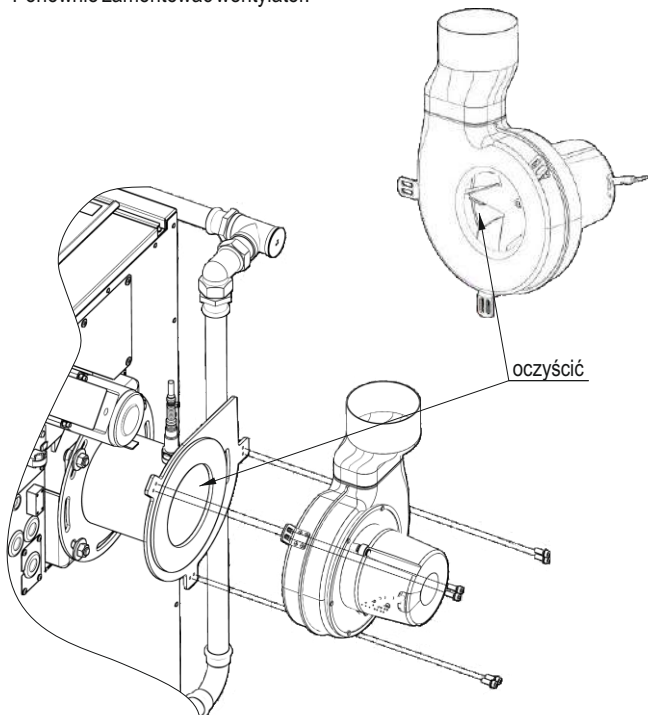
Rysunek 18. Sposób czyszczenia wentylatora wyciągowego.
