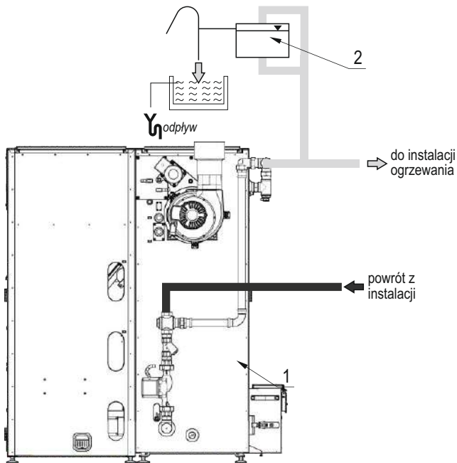
Rysunek 6. Przykładowy schemat zabezpieczeń kotła ALFA II: 1-kocioł; 2-otwarte naczynie wzbiorcze.
