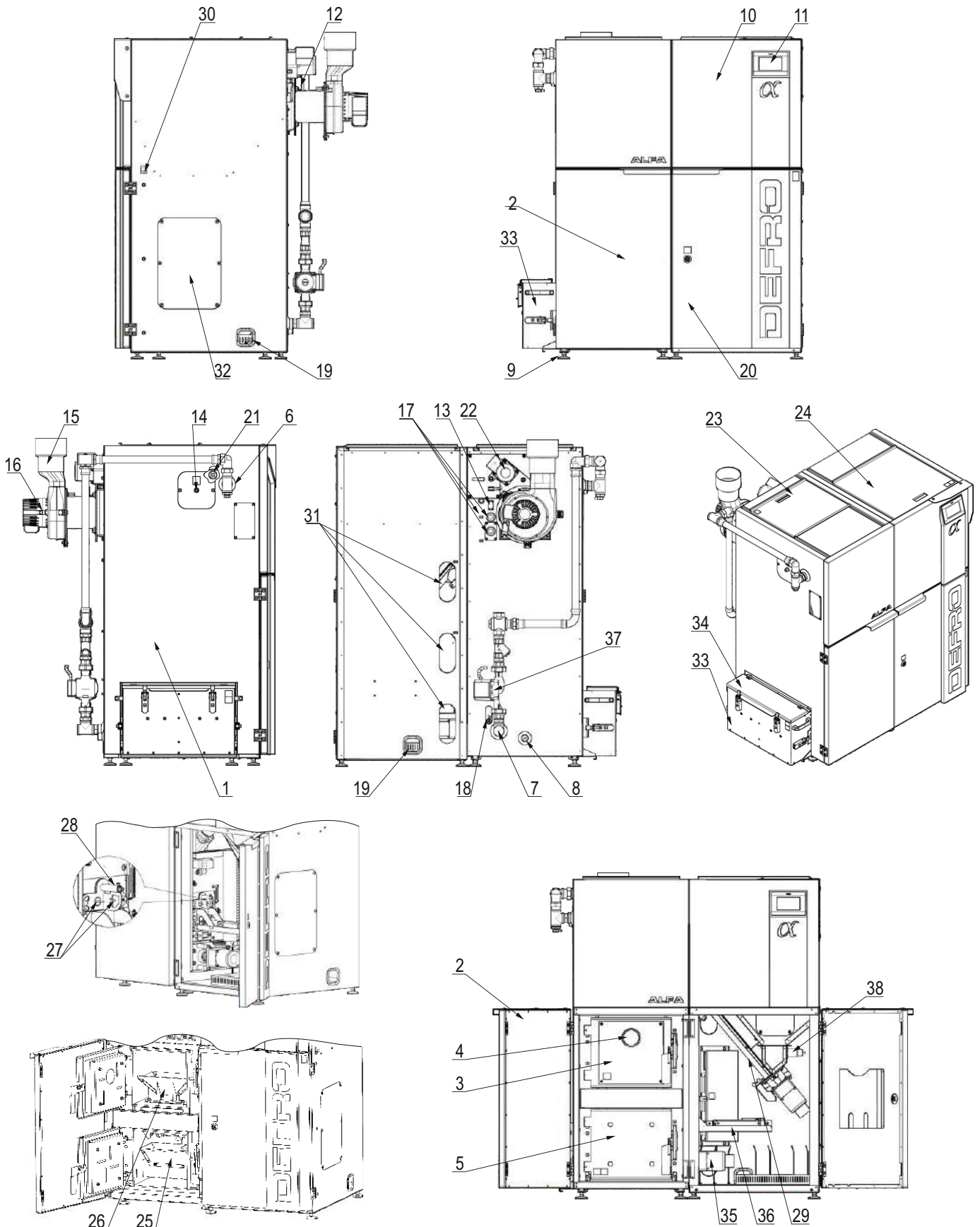
Rysunek 2. Podstawowe elementy kotłów ALFA II.
