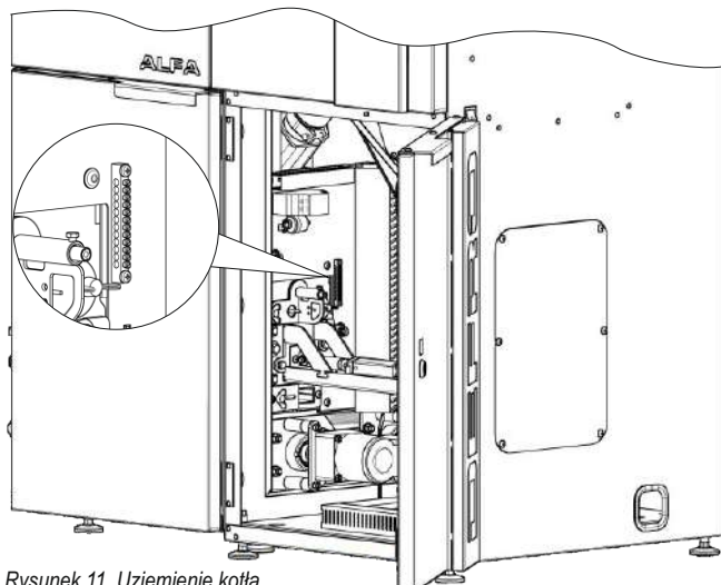
Rysunek 11. Uziemienie kotła.
