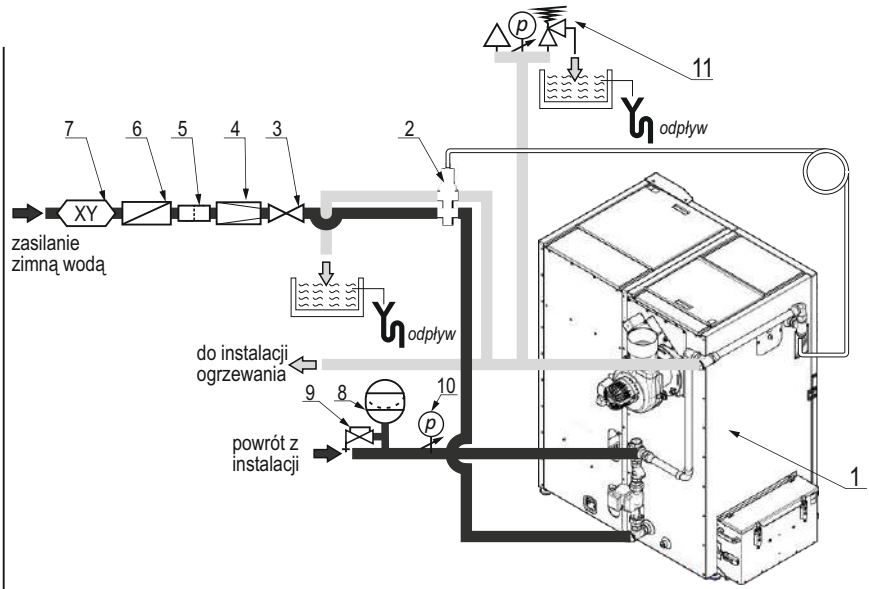
Rysunek 8. Przykładowy schemat zabezpieczeń kotła w układzie zamkniętym: 1-kocioł; 2-zabezpieczenie termiczne przed przegrzaniem /np. zawór 544/; 3-zawór kulowy; 4-reduktor ciśnienia; 5-filtr wody użytkowej; 6-zawór zwrotny; 7-zawór antyskażeniowy; 8-naczynie wzbiorcze; 9-zawór kółkowy; 10-manometr; 11-armatura bezpieczeństwa;
