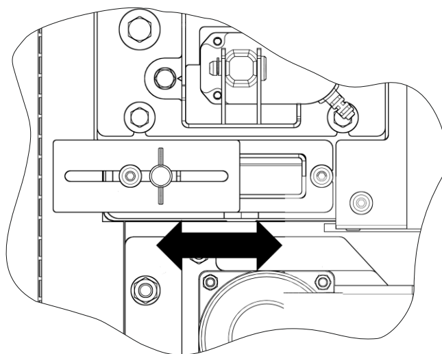
Rysunek 15. Fabryczne nastawy przepustnicy powietrza.
