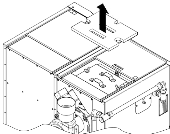
KROK 2. Usunąć izolację pokrywy wyczystnej.
