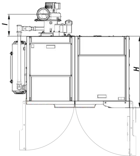
Rysunek 1. Podstawowe wymiary kotłów: ALFA II / ALFA II PLUS.
