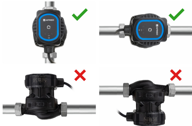
Rys. 1 Dopuszczalne pozycje montażowe pompy
