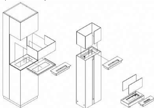
Obr. 5: Způsob montáže skel v biokrbch Sierra, Romeo, Galina
