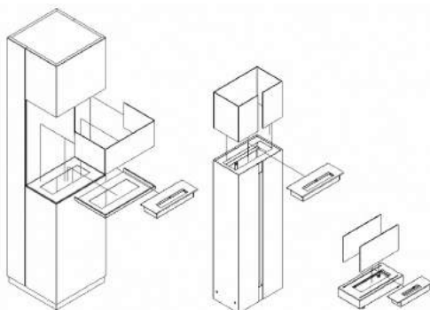
Dessin 3. Montage de la vitre dans les bio-cheminées Sierra, Romeo, Galina
