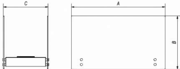
Рис. 8. Способ нанесения размеров био каминов Foxtrot, Galina, Hotel, Hotel Mini, Hotel Krzak, Hotel Mini Krzak, Linate
