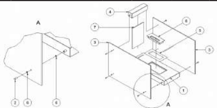
Obr. 4. Spôsob montáže biokozuba Linate
