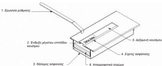
Εικ. 2 Δοχείο καύσης - διατομή
