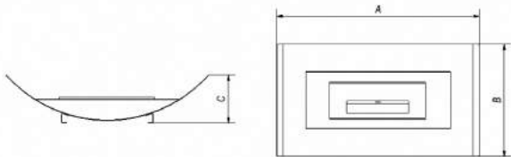
8 pav. Biožidinių „Foxtrot“, „Galina“, „Hotel“, „Hotel Mini“, „Hotel Krzak“, „Hotel Mini Krzak“, „Linate“ matavimo būdas
