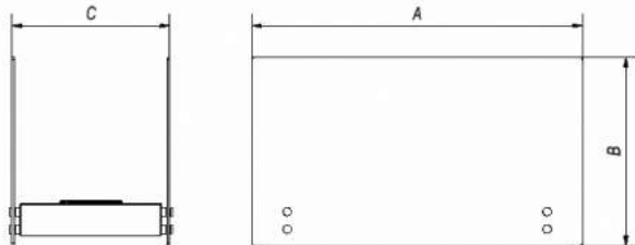
Obr. 8: Způsob dimenzování bikrbů Foxtrot, Galina, Hotel, Hotel Mini, Hotel Krzak, Hotel Mini Krzak, Linate
