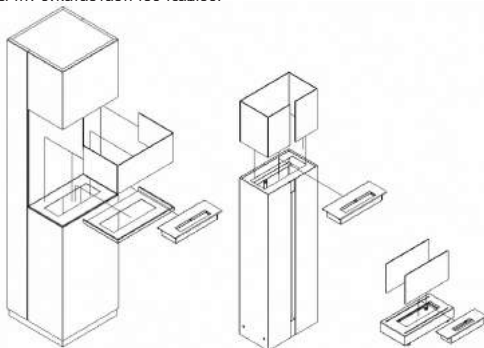
Εικ. 5 Τρόπος εγκατάστασης τζαμιού στα βιολογικά τζάκια Sierra, Romeo, Galina 6. Εγχειρίδιο χρήσης
