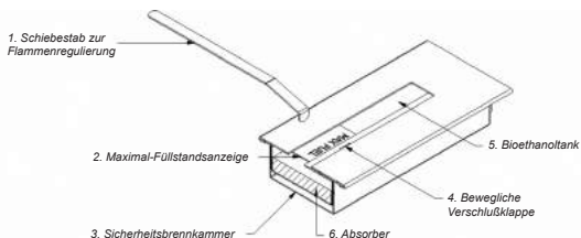
Zeichnung 2. Querschnitt der Sicherheitsbrennkammer
