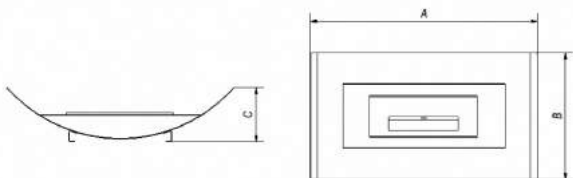
Dessin 9. Manière de mesurer les bio-cheminées „India“, „India Mini“, „India Max“, „Kilo“, „Misa“, „Misa Mini“ matavimo būdas
