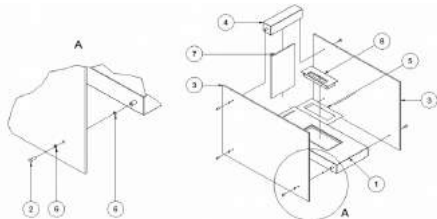
Zeichnung 4. Montageanleitung für den Biokamin Linatè
