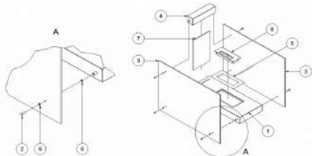
Obr. 4. Způsob montáže biokrbu Linat
