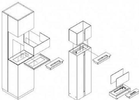
Fig. 5. Metodo di montaggio dei vetri nei biocaminetti Sierra, Romeo, Galina
