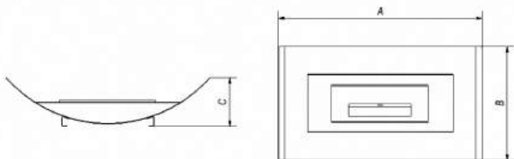
Zīm. 9. Iespēja izmēru atzīmēšana bio kamīniem India, India Mini, India Max, Kilo, Misa
