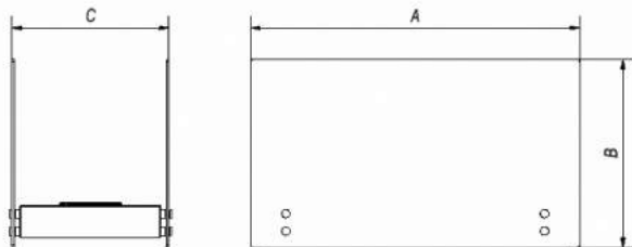
Zīm. 8 Iespēja izmēru atzīmēšana bio kamīniem Foxtrot, Galina, Hotel, Hotel Mini, Hotel Krzak, Hotel Mini Krzak, Linate
