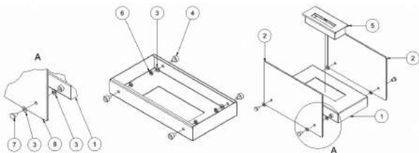
Zeichnung 3. Montageanleitung für die Biokamine: Hotel, Mini, Bush Hotel, Hotel Mini Busch
