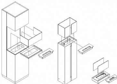
5.sz.kép: A Sierra, Romeo, Galina bio kandallók üvegei szerelésének módja
