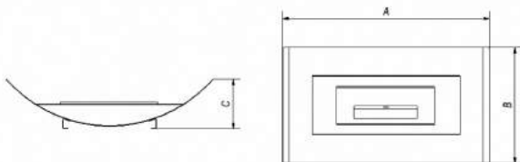
9.sz.kép: Galina India, India Mini, India Max, Kilo, Misa, Misa Mini bio kandallók méretei
