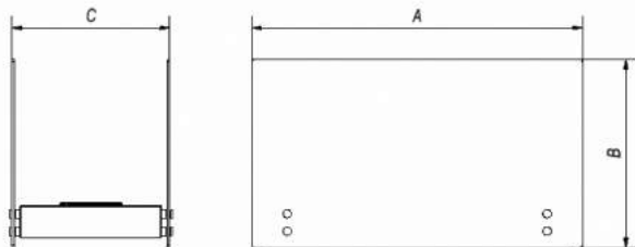
8.sz.kép: Foxtrot, Galina, Hotel, Hotel Mini, Hotel Krzak, Hotel Mini Krzak, Linate bio kandallók méretei
