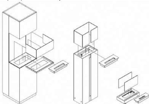
Obr. 5: Spôsob montáže skiel v biokozuboch Sierra, Romeo, Galina
