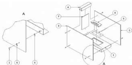
Рисунок 4. Способ монтажа био камина Linate
