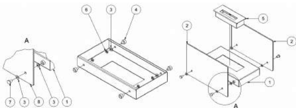
Εικ. 3 Τρόπος εγκατάστασης βιολογικών τζακιών: Hotel, Hotel Mini, Hotel Krzak, Hotel Mini Krzak
