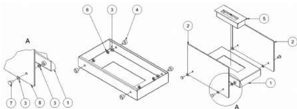
Slika 3. Način montaže bio-kaminov: Hotel, Hotel Mini, Hotel Krzak, Hotel Mini Krzak
