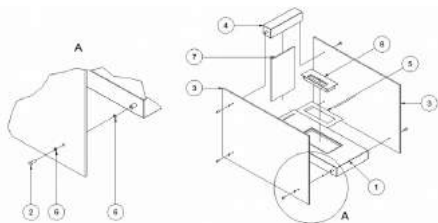
4. attēls. Stikla montāža biokamīnos Linatē
