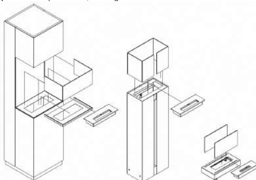
Slika 5. Način montaže stekel v bio-kaminih Sierra, Romeo, Galina
