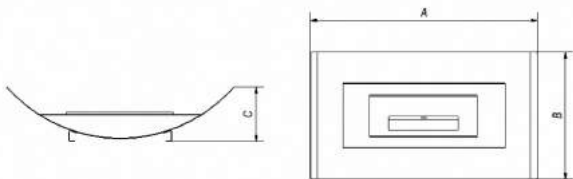
Zeichnung 9. Ausmaß von India, India Mini, India Max, Kilo, Misa, Misa Mini
