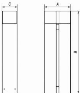
10.sz.kép: Sierra, Romeo bio kandallók méretei
