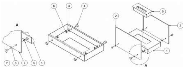
Obr. 3. Způsob montáže biokrbů: Hotel, Hotel Mini, Hotel Krzak (Keř), Hotel Mini Krzak (Keř)
