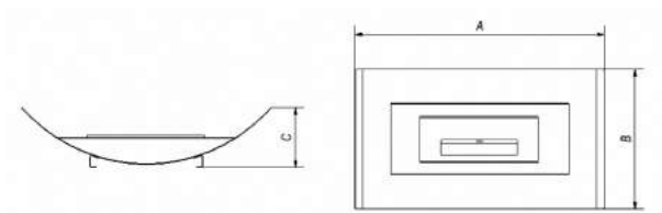
Obr. 9: Spôsob dimenzovania biokozubov India, India Mini, India Max, Kilo, Misa, Misa Mini
