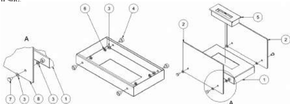
Рисунок 3. Способ монтажа био каминов : Hotel, Hotel Mini, Hotel Krzak, Hotel Mini
