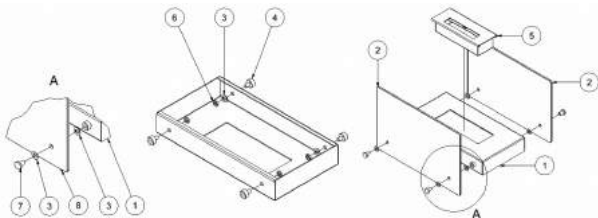
3.sz.kép: Hotel, Hotel Mini, Hotel Krzak (Keř), Hotel Mini Krzak (Keř) bio kandallók szerelésének módja
