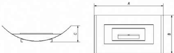
Εικ. 8 Τρόπος μέτρησης διαστάσεων των βιολογικών τζακιών India „India Mini“, „India Max“, „Kilo“, „Misa“, „Misa Mini“
