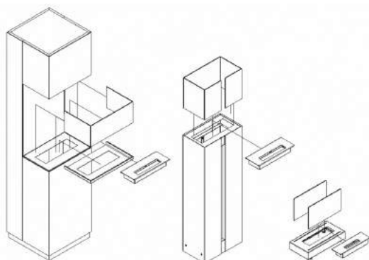
Рисунок 5. Способ монтажа стекла в био-каминах Sierra, Romeo, Galina
