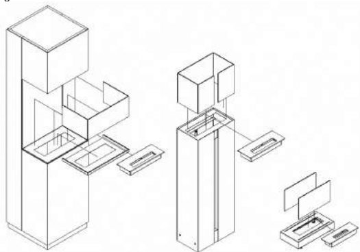
Zeichnung 5. Anleitung zum Einbau des Schutzglases der Biokamine Sierra, Romeo, Galina
