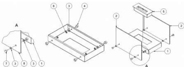
3. attēls. Stikla montāža biokamīnos Hotel, Mini, Bush Hotel, Hotel Mini Busch
