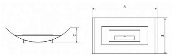
Fig. 9. Metodo di dimensionamento dei biocaminetti India, India Mini, India Max, Kilo, Misa, Misa Mini
