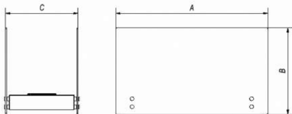
Εικ. 8 Τρόπος μέτρησης διαστάσεων των βιολογικών τζακιών „Foxtrot“, „Galina“, „Hotel“, „Hotel Mini“, „Hotel Krzak“, „Hotel Mini Krzak“, „Linat“
