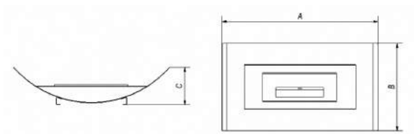
Рис. 9. Способ нанесения размеров био каминов India, India Mini, India Max, Kilo, Misa, Misa Mini
