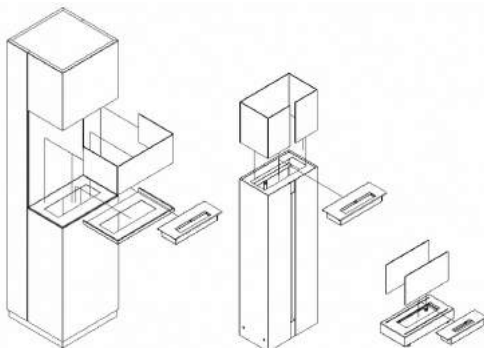
5 pav. Biožidinių „Sierra“, „Romeo“ ir „Galina“ stiklų montavimo būdas
