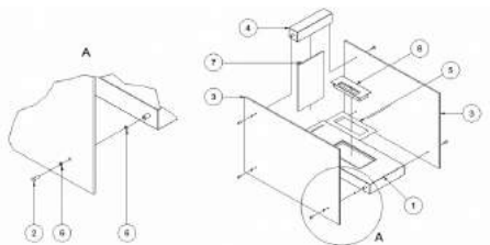
Dibujo 4. Modo de instalación de biochimenea Linat
