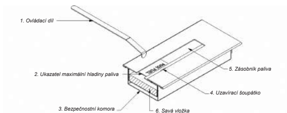
Obr. 2: Nádoba na biopalivo – průřez
