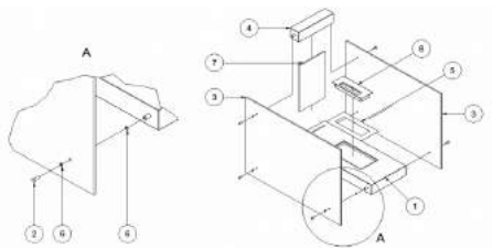
4 pav. Biožidinio „Liniate“ įrengimo būdas
