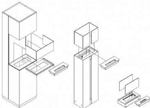
5. attēls. Stikla montāža biokamīnos Sierra, Romeo, Galina
