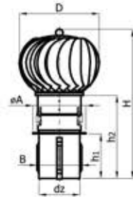
10. Podstawa rurowa - nieotwierana -B-S
