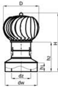
7. Podstawa z kołnierzem zamykającym ocieplenie - otwierana -B-K-U
