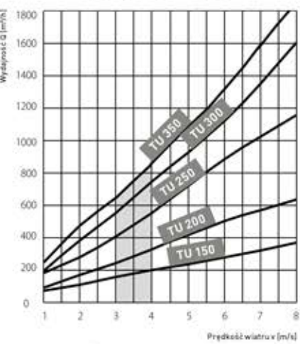
Wykres wydajności obrotowych nasad kominowych TURBOWENT w zależności od prędkości wiejącego wiatru bez uwzględnienia wysokości kominu. [*1[m/s]=3,6[km/h]].
