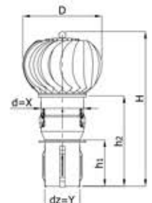
14. Podstawa redukcyjna wciskana -X/Y-...PTU
