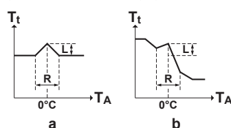
a Bezwzględna żądana T_{\text{zasil}} b Zależna od pogody żądana T_{\text{zasil}}
