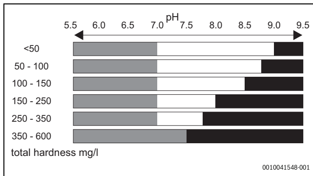
Rys. 13 Jakość wody
