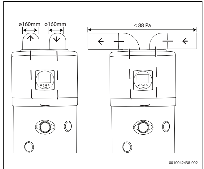
Rys. 11 Drugi osobny przewód powietrza
