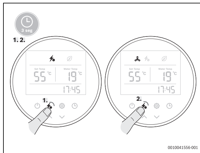
Rys. 24 Ustawianie trybu tylko podgrzewacza elektrycznego
