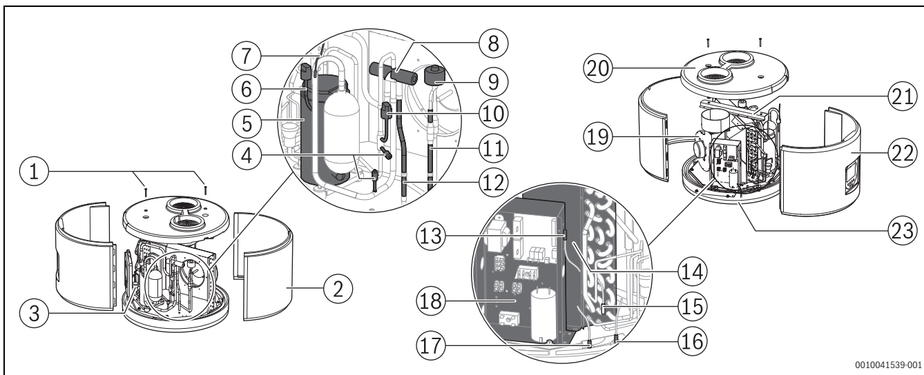
Rys. 4 Przegląd produktu
