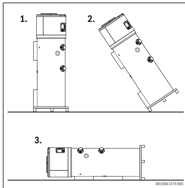
Rys. 5 Pochylenie urządzenia
