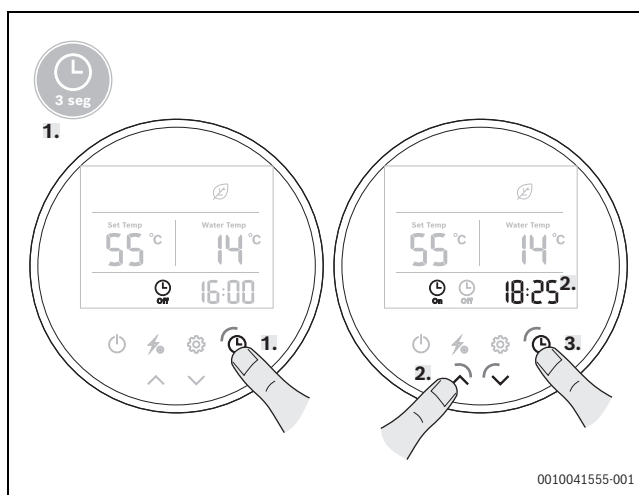
Rys. 20 Ustawianie zegara sterującego
