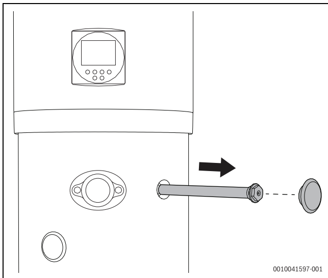
Rys. 31 Wymywanie anody magnezowej
