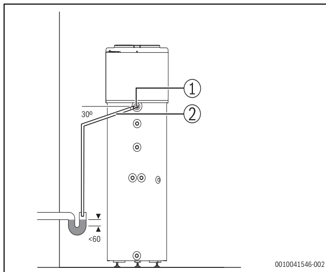
Rys. 12 Podłączanie odprowadzenia kondensatu
