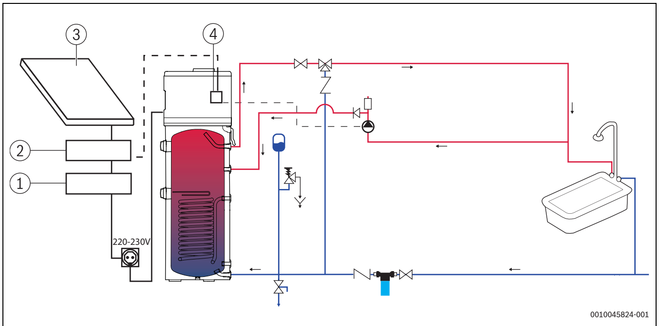
Rys. 37 Recyrkulacja
