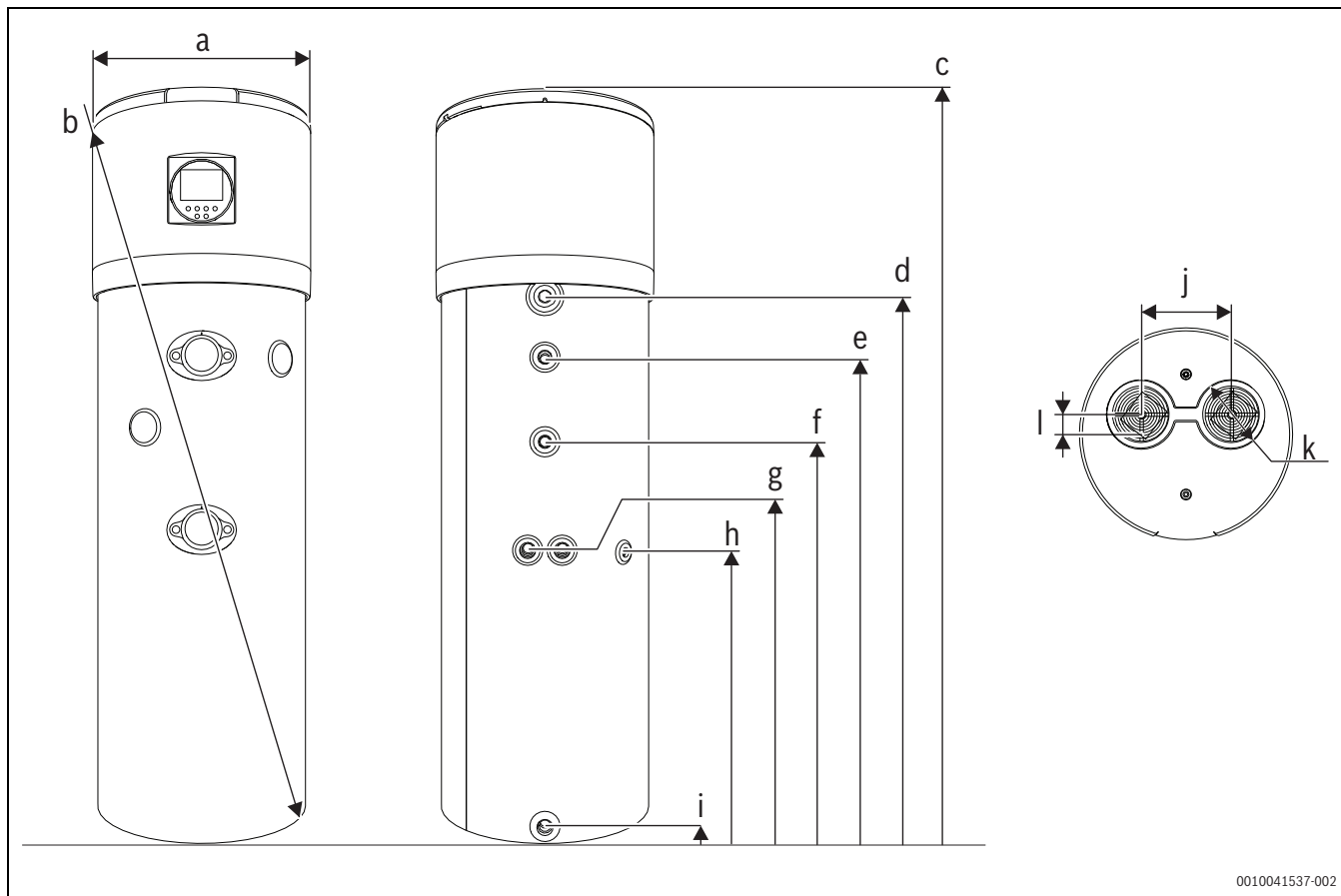
Rys. 2 Wymiary urządzenia
