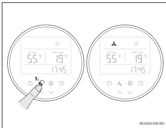
Rys. 26 Ustawianie trybu wentylacji za pomocą wentylatora
