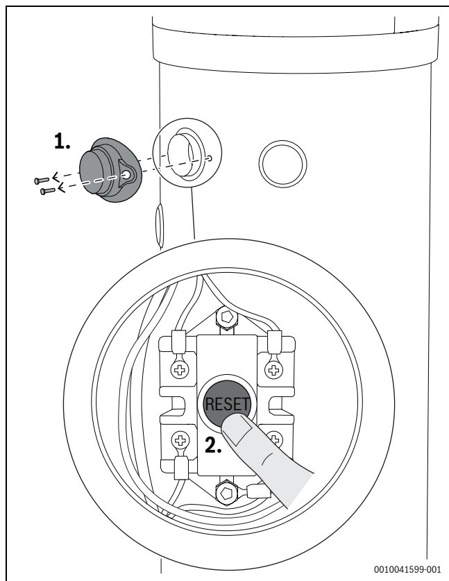
Rys. 32 Resetowanie termostatu
