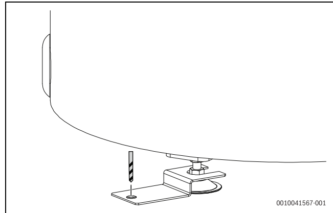
Rys. 8 Wspornik mocujący
