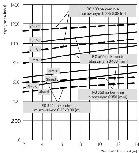
Wykres wydajności samonastawnych nasad kominowych ROTOWENT Ø350 i Ø400 dla komin blaszanych i murowanych, dla dwóch prędkości wiatru 3 i 4 [m/s].
