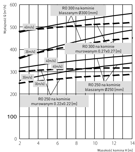
Wykres wydajności samonastawnych nasad kominowych ROTOWENT Ø250 i Ø300 dla komin blaszanych i murowanych, dla dwóch prędkości wiatru 3 i 4 [m/s].
