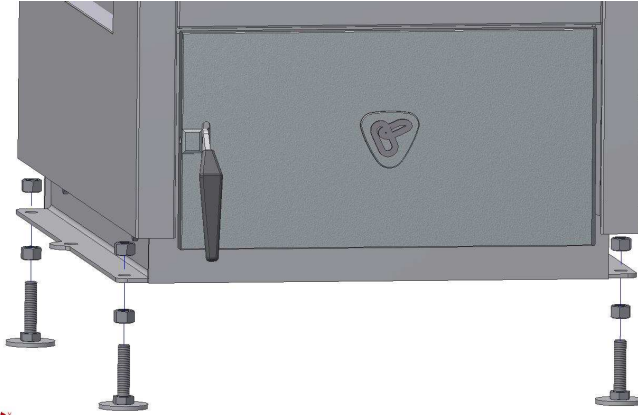
Montaż nastawnych nóg kotła
