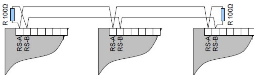
Rysunek 9: Przykładowy schemat prawidłowego połączenia interfejsu RS485
