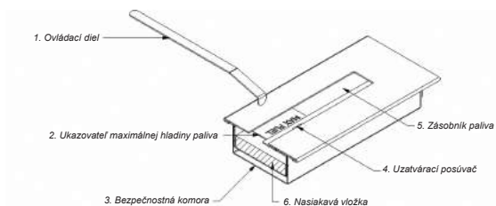
Obr. 2: Nádoba na biopalivo – prierez
