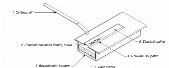
Obr. 2: Nádoba na biopalivo – průřez
