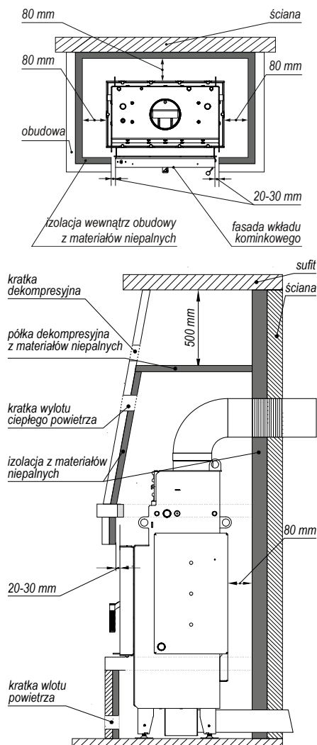
Rysunek 8. Przykładowa zabudowa wkładu kominkowego.
