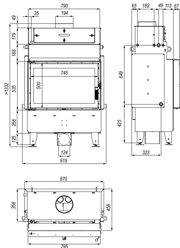
Rysunek 3. Rzuty z wymiarami wkładu kominkowego NAVI ME.
