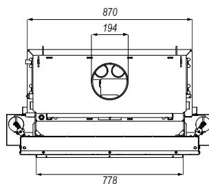
Rysunek 7. Rzuty z wymiarami wkładu kominkowego NAVI ME G.
