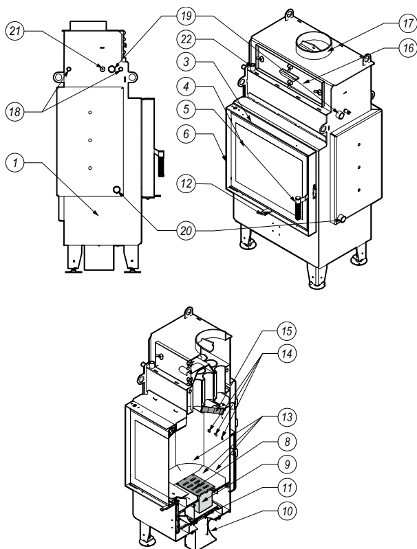
Rysunek 1. Budowa wkładu kominkowego NAVI.
