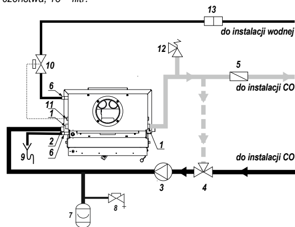
Rysunek 13. Schemat przykładowego podłączenia zespołu wodnego kominika NAVI z systemem grzewczym w układzie zamkniętym.
