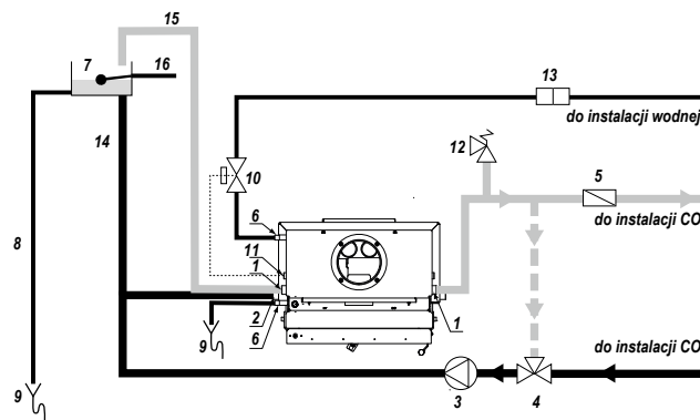
Rysunek 12. Schemat przykładowego podłączenia zespołu wodnego kominika NAVI z systemem grzewczym w układzie otwartym.
