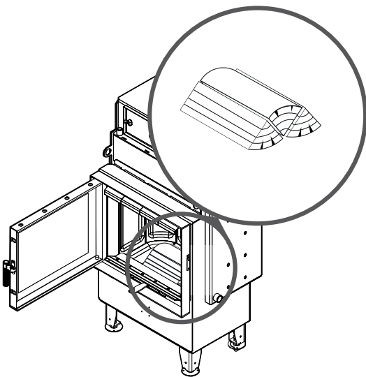
Rysunek 14. Sposób ułożenia paliwa podczas rozpali
