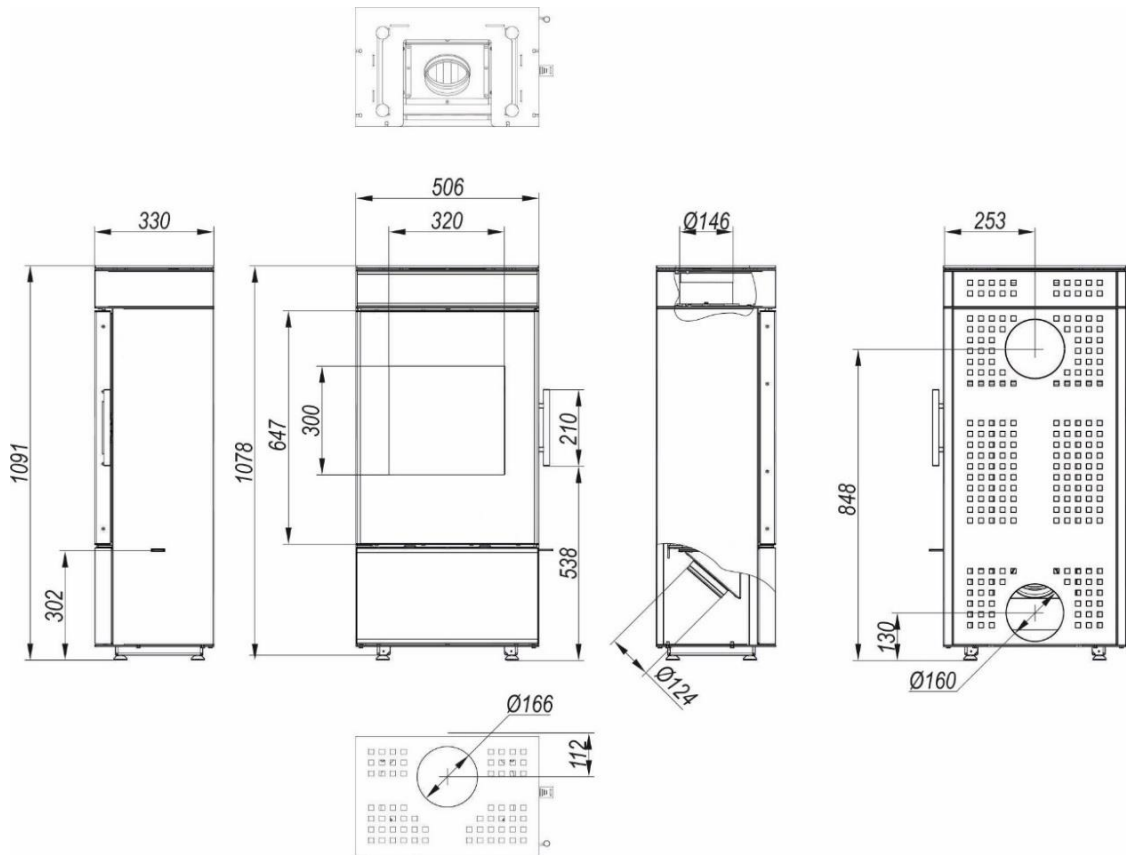
Rysunek 7. Wymiary (w mm) ogrzewacza DEFRO HOME CUBE MINI
