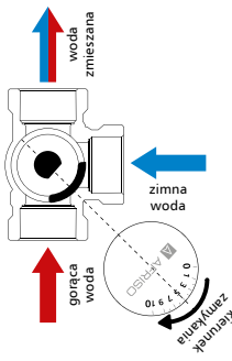
Rys. 5. 3-drogowy, pozycja 2.
