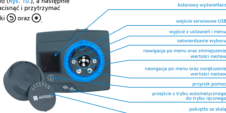
Rys. 10. Opis regulatora.
