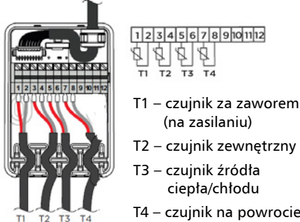
Rys. 9. Kostka podłączeniowa regulatora ARC 345 ProClick.
